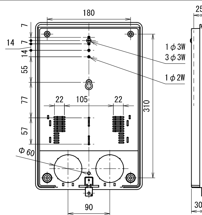
基台 (取付板)
